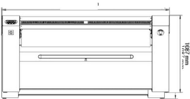
Vue avant
